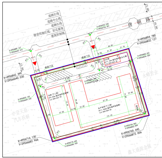
总平面图
