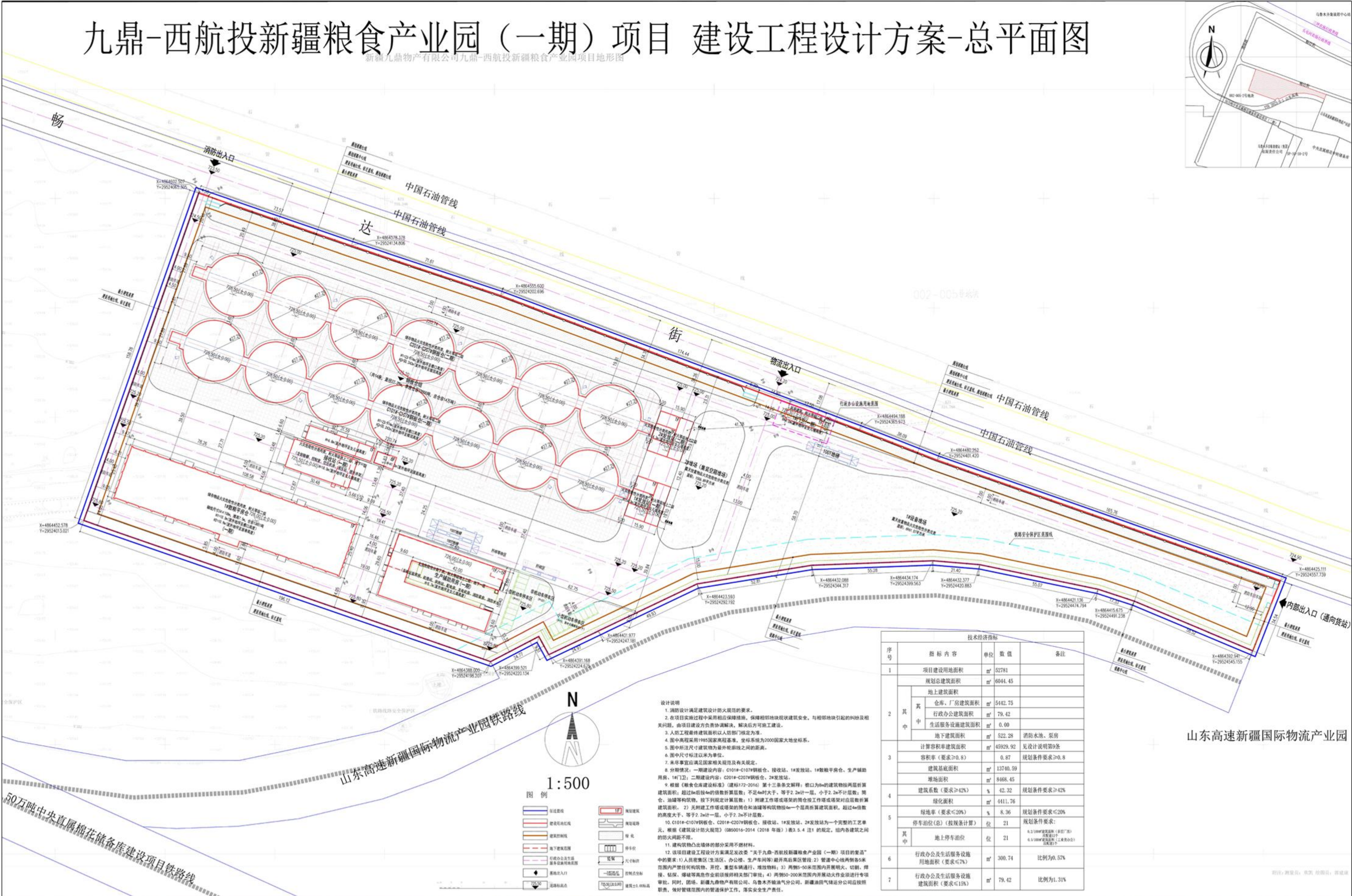
总平面图
