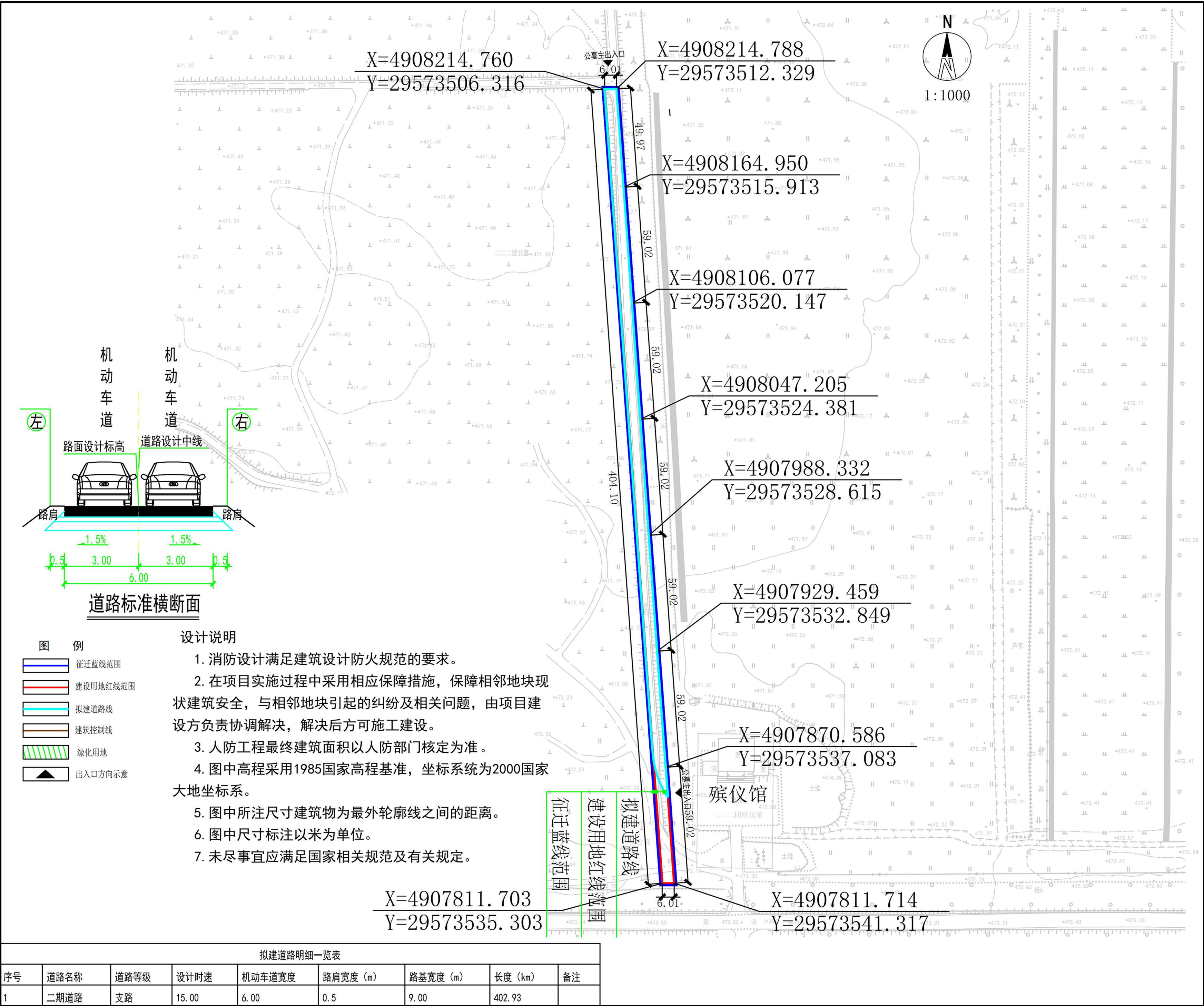
总平面图
