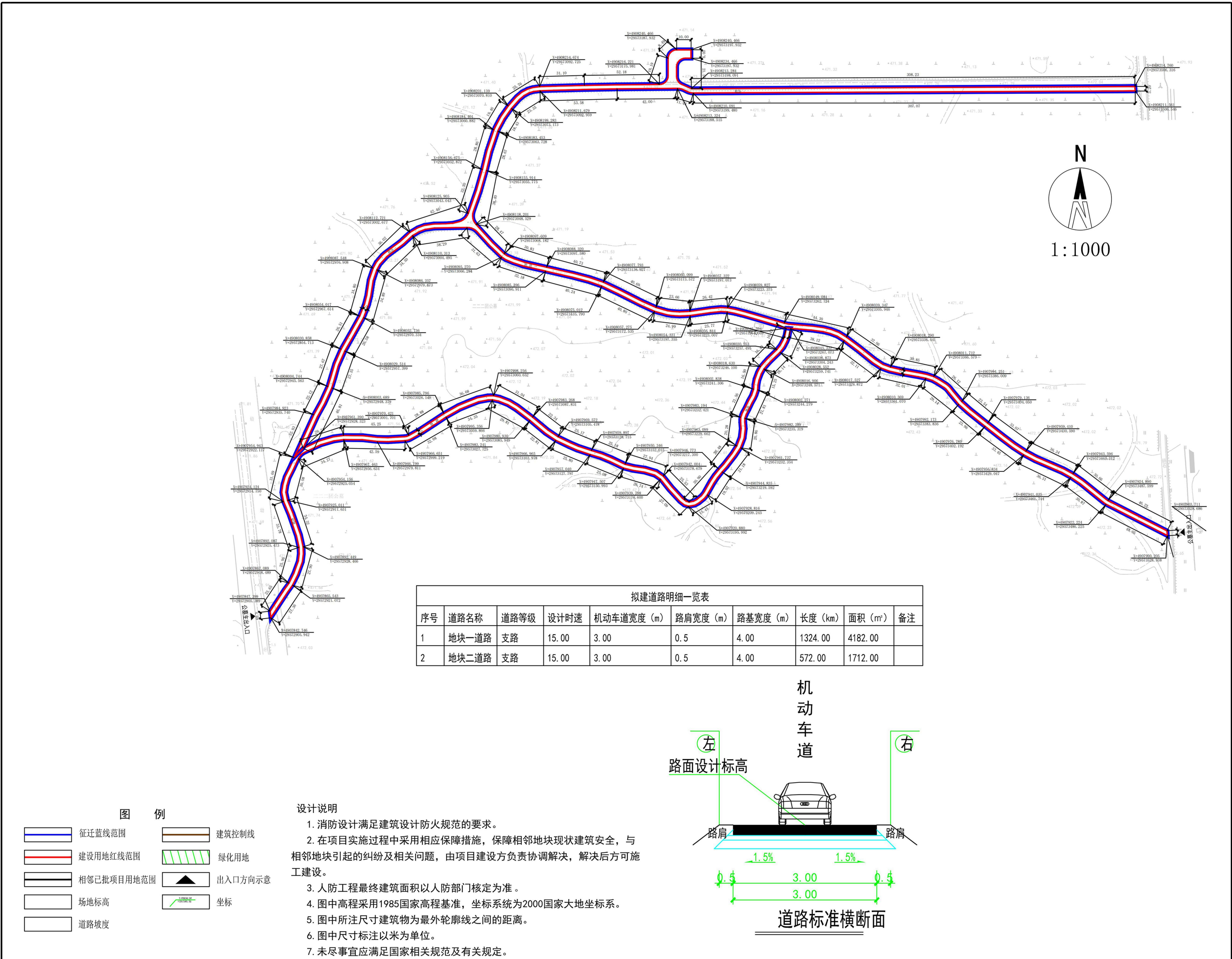
总平面图
