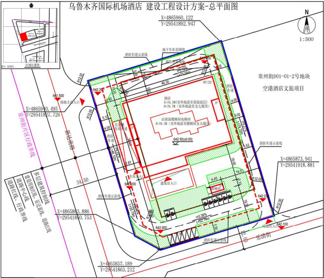
总平面图
